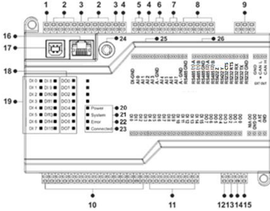
Şekil 4 GA2 Kartı Klemens ve Fiziksel Arayüzü
