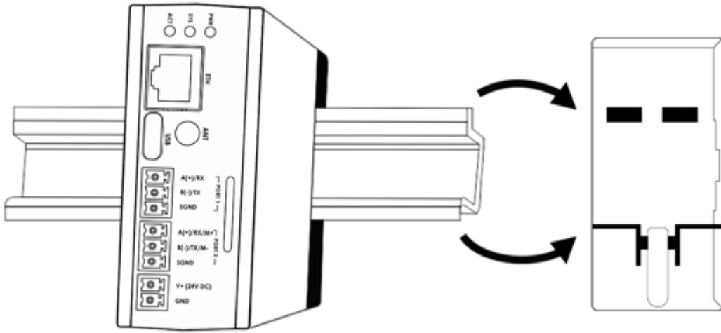
Şekil 2 Montaj Bilgileri
