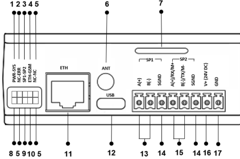
Şekil 1 Klemens ve Fiziksel Arayüzler
