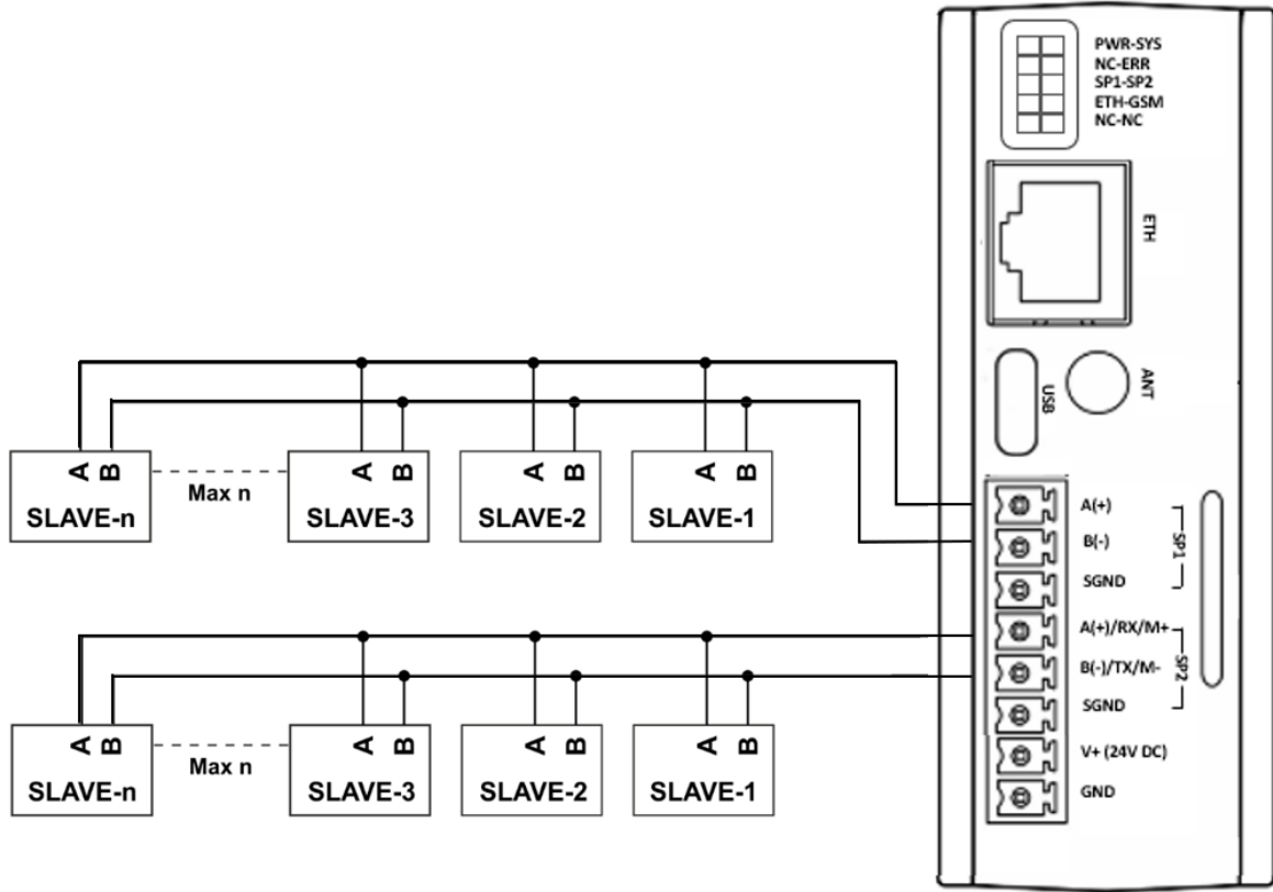
Şekil 5 RS485 Giriş Bağlantı Şeması
