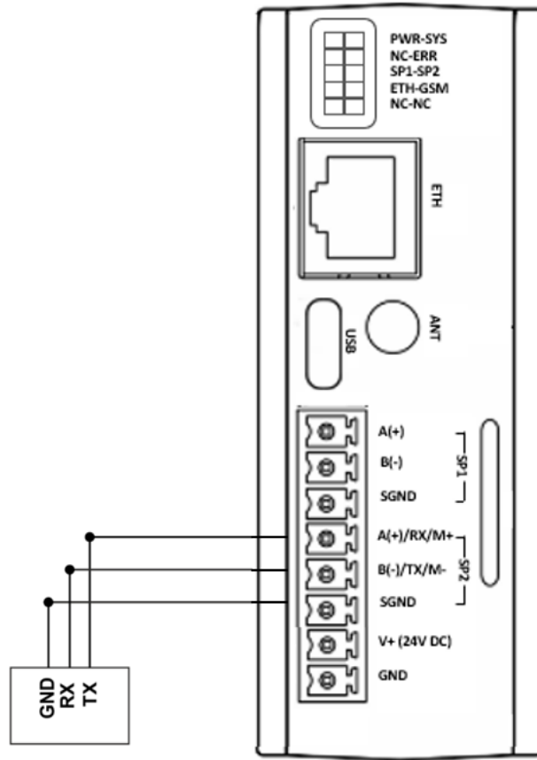
Şekil 6 RS232 Giriş Bağlantı Şeması
