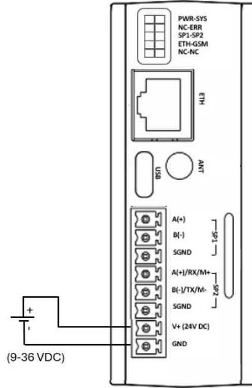
Şekil 4 Güç Bağlantı Şeması
