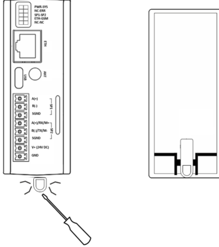
Şekil 3 Demontaj Bilgileri
