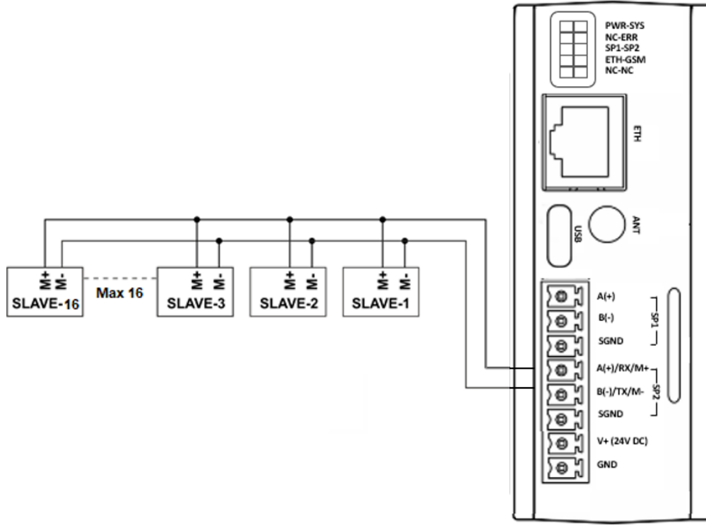
Şekil 6 M-BUS Portu Giriş Bağlantı Şeması
