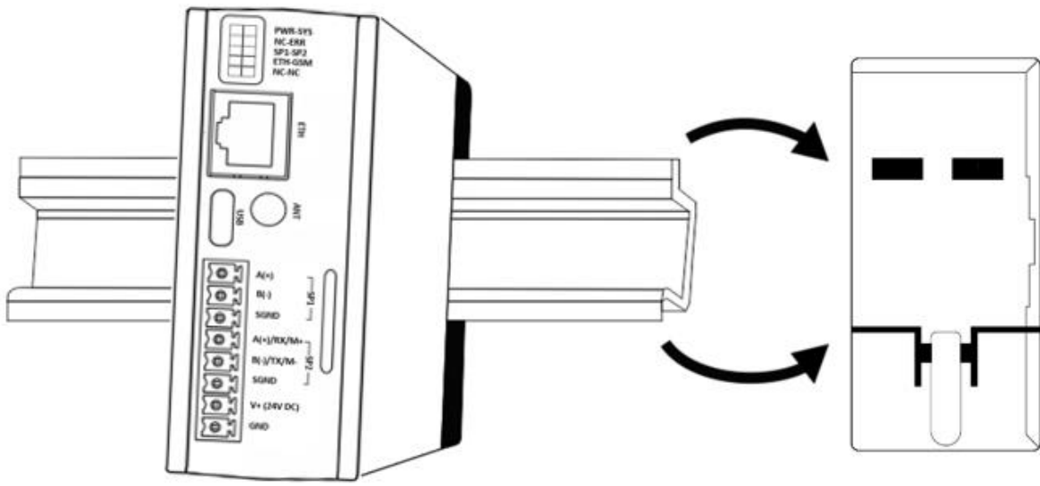
Şekil 2 Montaj Bilgileri
