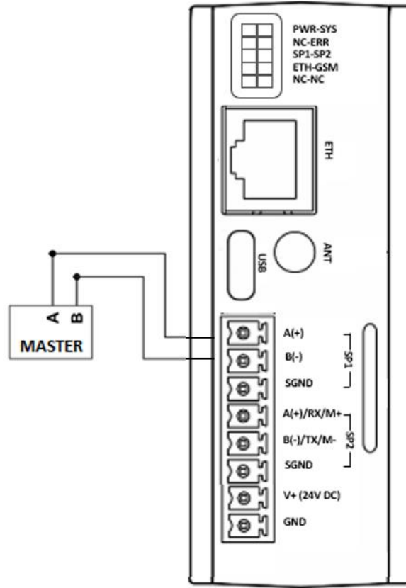
Şekil 5 RS485 Portu Giriş Bağlantı Şeması
