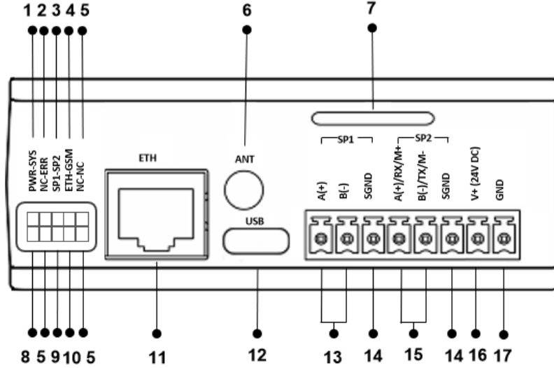
Şekil 1 GC1 Kartı Klemens ve Fiziksel Arayüzler
