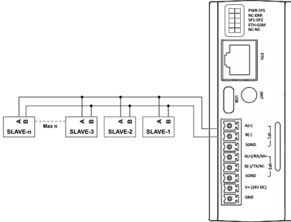
Şekil 5 RS485 Giriş Bağlantı Şeması
