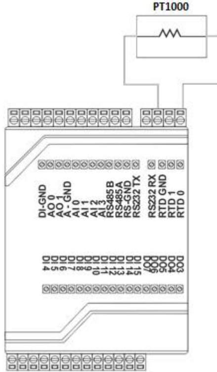
Şekil 13 RTD Giriş Bağlantı Şeması
